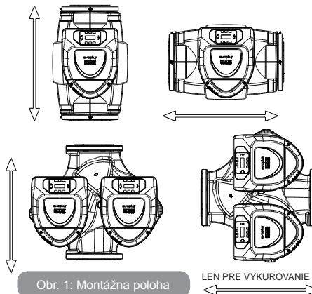
Obr. 1: Montážna poloha
