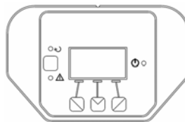
Figura 10: Panou de control
