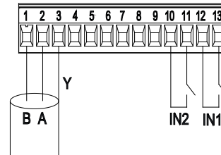
Εικόνα 7: Αφαιρούμενη κλέμμα 13 πόλων: ψηφιακές εισοδοι και MODBUS
