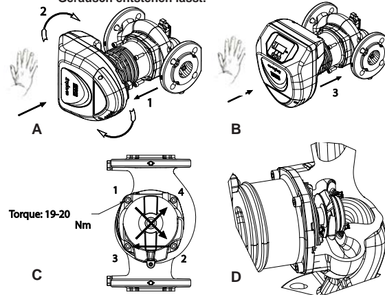
Abbildung 2: Montageanleitungen für Motorkopf
