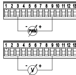
Obr. 8: Vyberateľná 13-pólová svorkovnica: vstupy 0-10V a PWM
