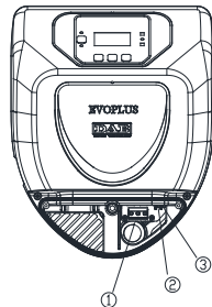
Figura 4: Conexiones eléctricas (frente)
