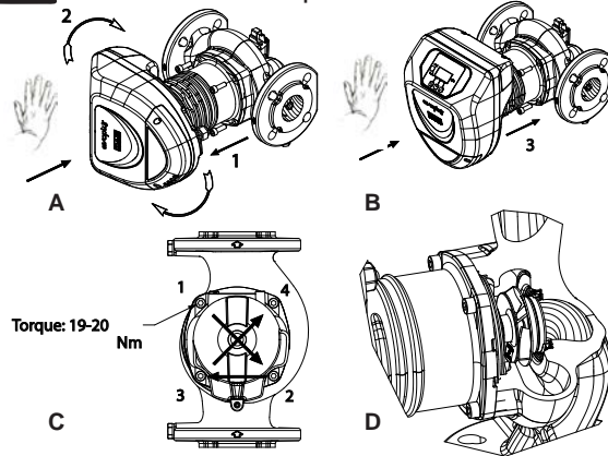
Figura 2: Instrucciones de montaje cabezales del motor
