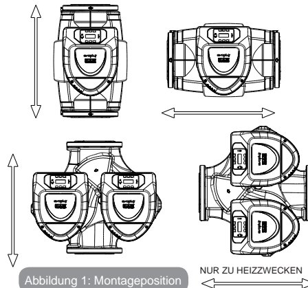
Abbildung 1: Montageposition
