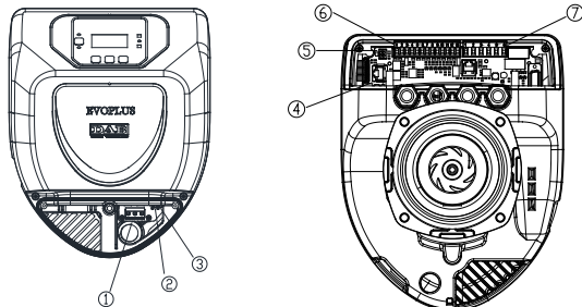
Figura 4: Conexiuni electrice (față)
