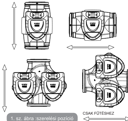
1. sz. ábra :szerelési pozíció
