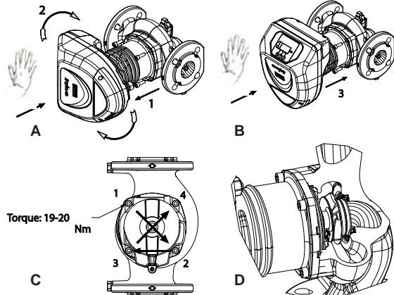
Resim 2: Motor kafaları montaj talimatları
