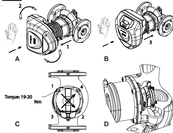
Figura 2: Instruções de montagem cabeças motor
