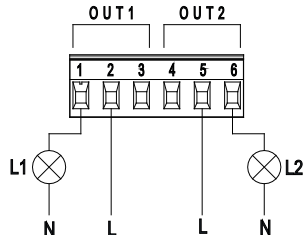
Εικόνα 9: Αφαιρούμενη κλέμμα 6 πόλων: παράδειγμα σύνδεσης εξόδων
