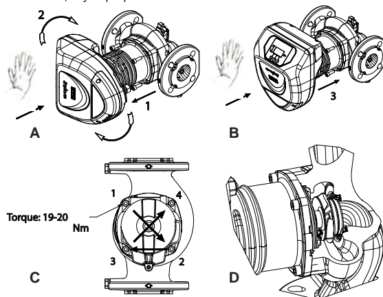
Фиг. 2: Инструкции за монтаж на моторната глава
