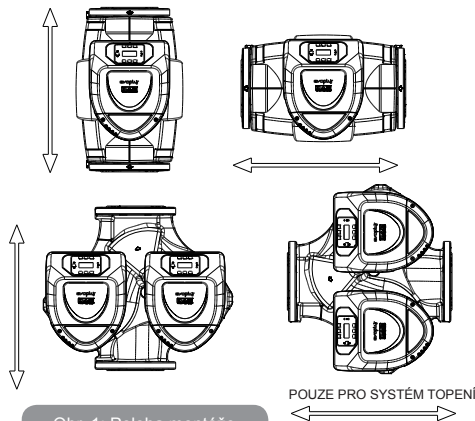
Obr. 1: Poloha montáže
