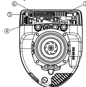
Attēls 5: Elektriskie savienojumi (aizmuģurē)
