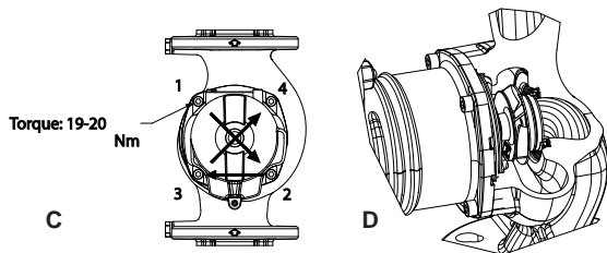
2. sz. ábra: Motortestek szerelési utasítása
