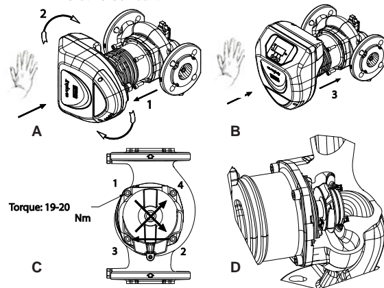
Afbeelding 2: Montage-instructies motorblokken
