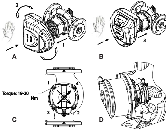
Kuv. 2: Moottorin päiden asennusohjeet
