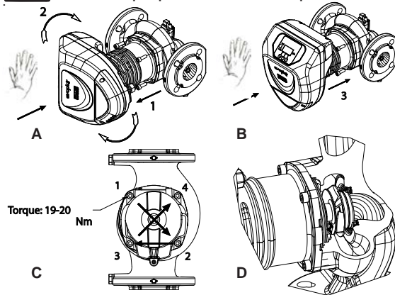
Obr 2: Návod na montáž hlav motoru
