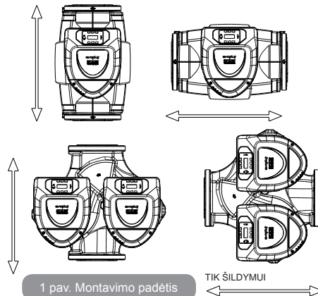
1 pav. Montavimo padėtis
