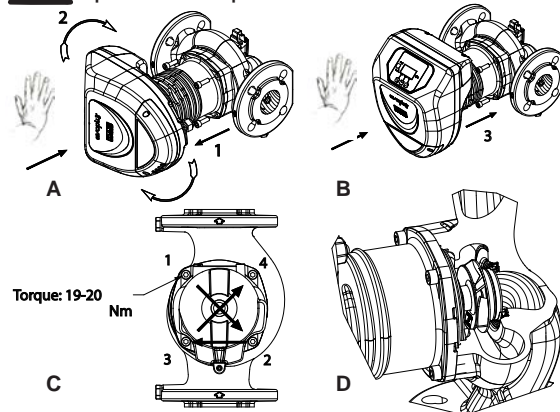
Figure 2: Instrucțiuni de montare capete motor
