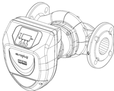
Attēls 3: Uzstādīšana uz horizontāliem cauruļvadiem
