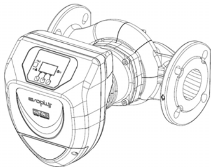
Figura 3: Instalación en tuberías horizontales
