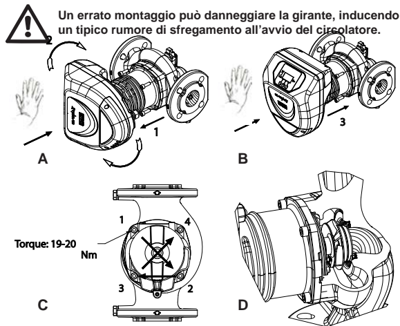
Figura 2: Istruzione di montaggio teste motore
