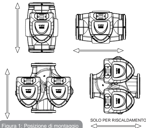
Figura 1: Posizione di montaggio
