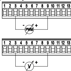
Εικόνα 8: Αφαιρούμενη κλέμμα 13 πόλων: είσοδοι 0-10V και PWM
