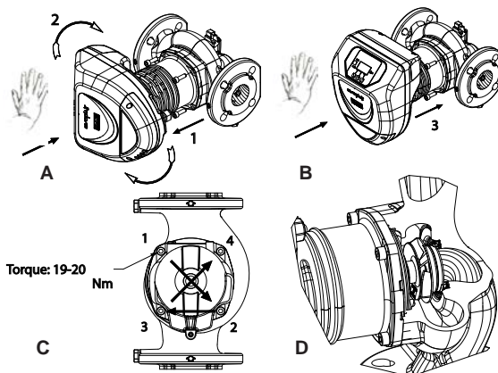
Obr. 2: Návod na montáž hláv motora
