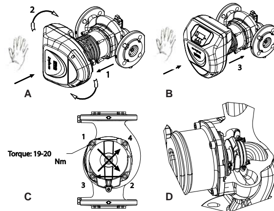
Fig 2: Monteringsanvisningar för motorhuvud
