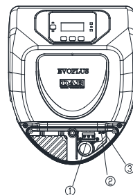
Abbildung 4: Elektroanschlüsse (Frontseite)
