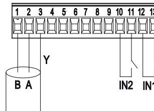
Afbeelding 7: Uittrekbaar 13-polig klemmenbord: digitale ingangen e MODBUS
