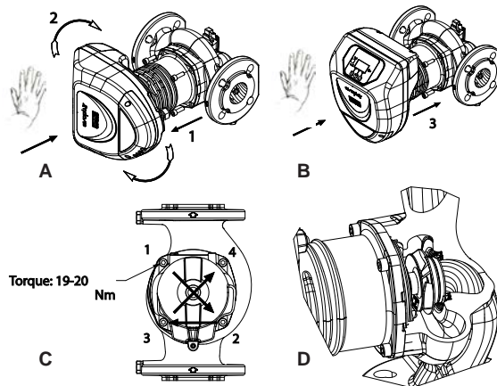
Attēls 2: Dzinēja galvīņu montāžas instrukcijas
