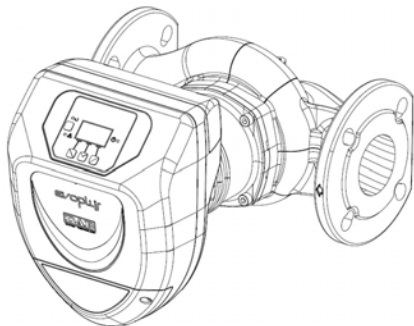
Фигура 3: Монтаж на хоризонтален тръбопровод
