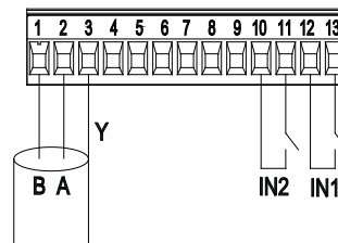
Figura 7: Morsettieria estraibile 13 poli: ingressi digitali e MODBUS
