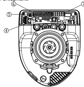
Abbildung 5: Elektroanschlüsse (Rückseite)
