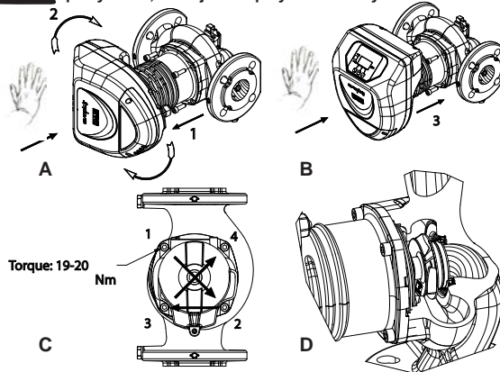
Rys. 2: Instrukcja montażu głowicy silnika
