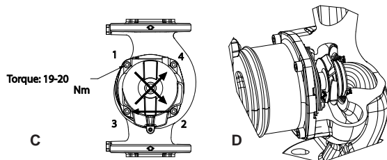
Εικόνα 2: Οδηγίες για την συναρμολόγηση των κεφαλών του κινητήρα
