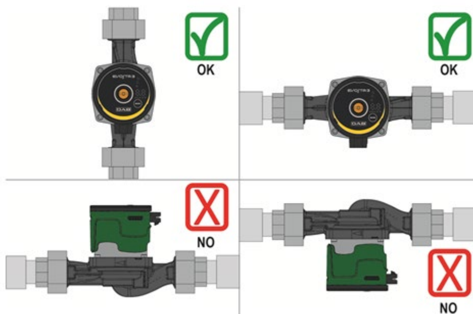
Obrázek.3: Poloha montáže
