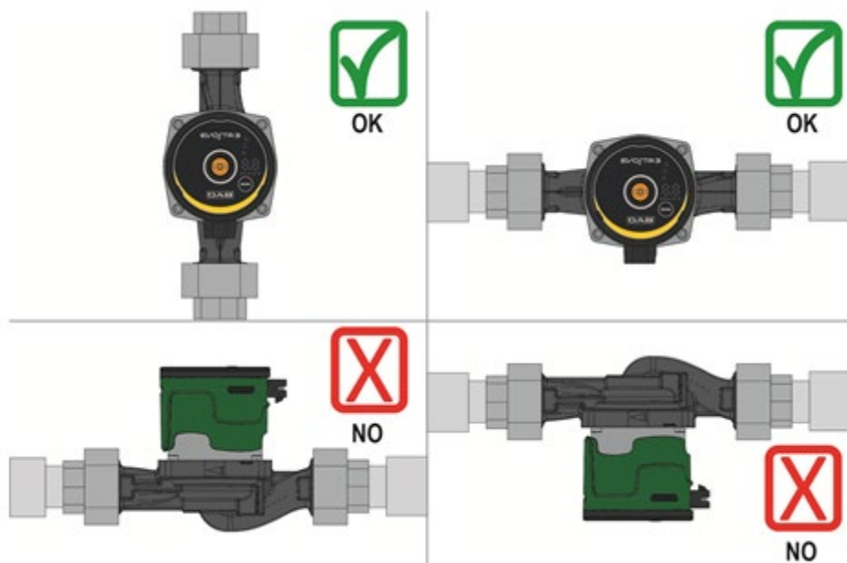
Slika 3: Vgradni položaji
