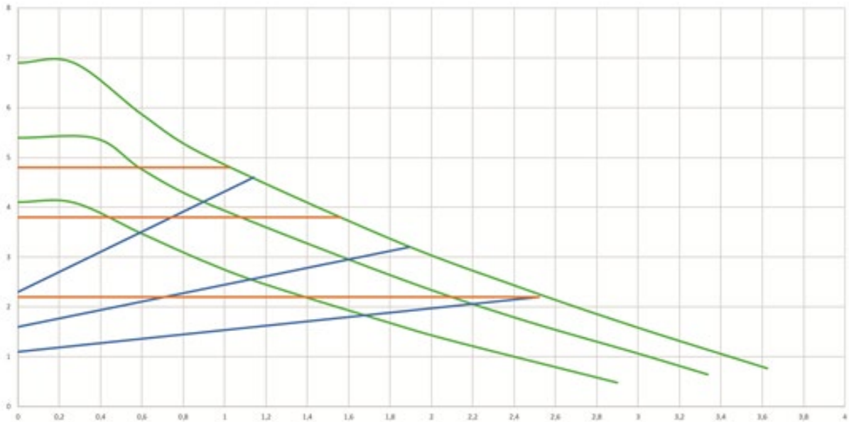
EVOSTA2 40-70/XXX
