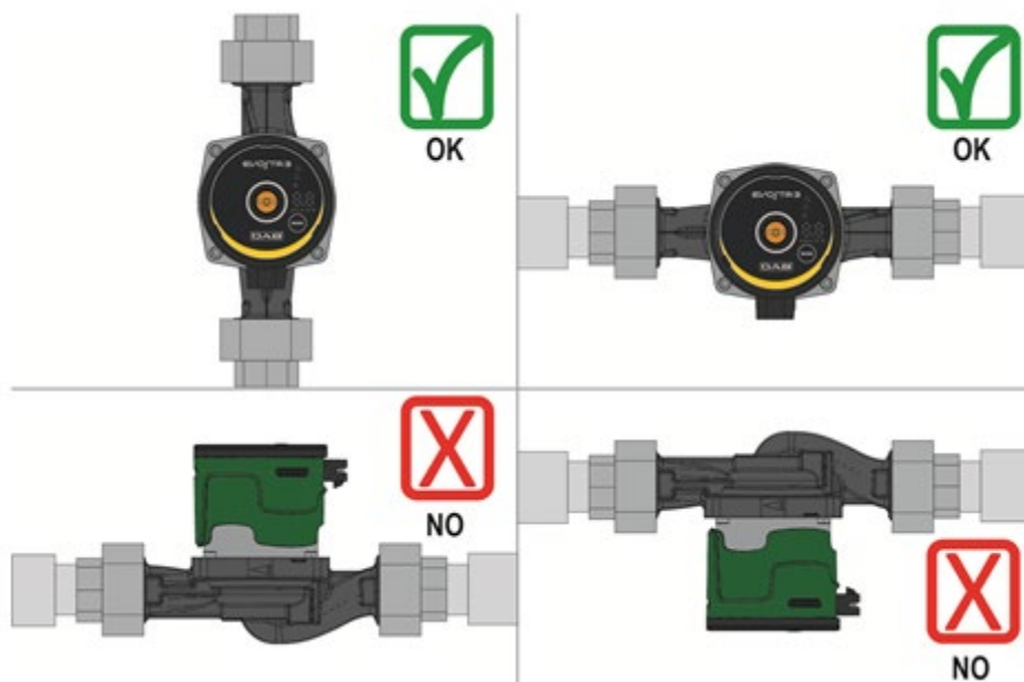
Obrázok 3: Montážna poloha
