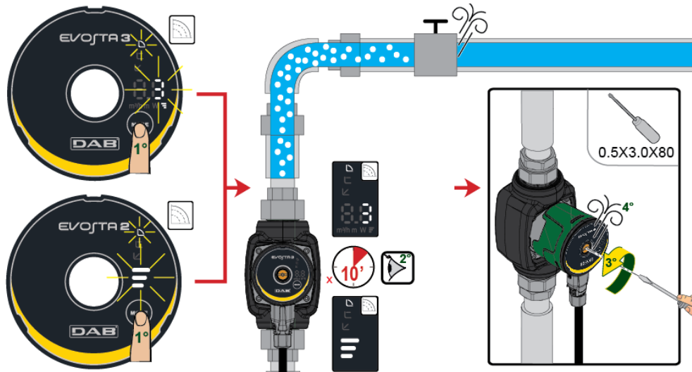
Figura 8: Aerisirea pompei
