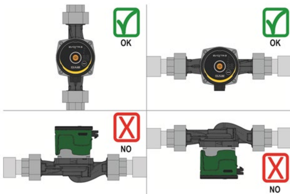
Abb. 3: Montageposition
