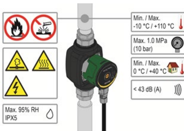
1. ábra: Szivattyúzott folyadékok, figyelmeztetések és működési feltételek
