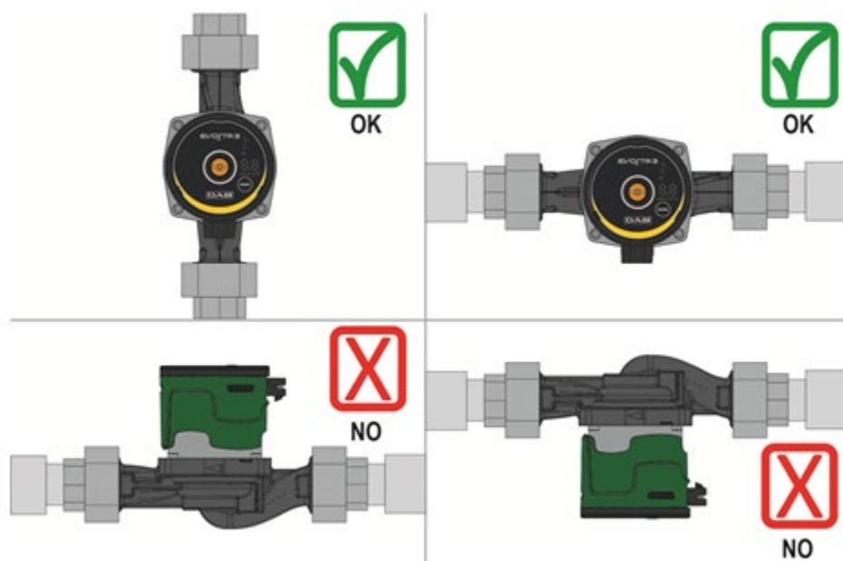
Fig 3: Monteringsläge
