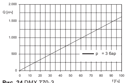
Рис. 24 DMX 770-3
