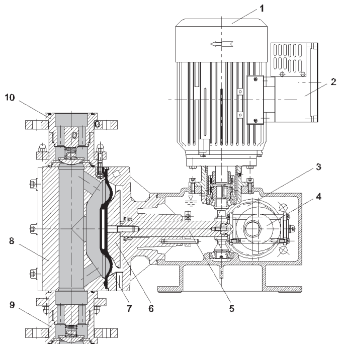
1-сур. DMX 227
