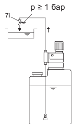
Рис. 10 Установка с клапаном поддержания давления
