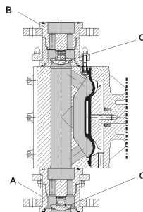
12-сур. Сорғыш және айдау желісін қосу
