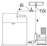
Рис. 9 Установка с предохранительным клапаном
