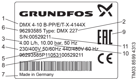
2-сур. DMX түрлі сорғылардың фирмалық тақтайшасы
