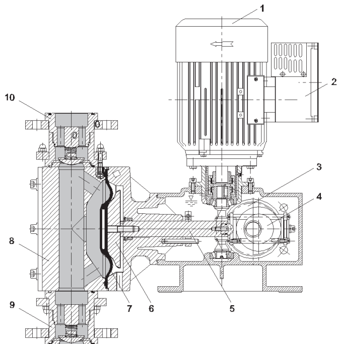
Рис. 1 DMX 227
