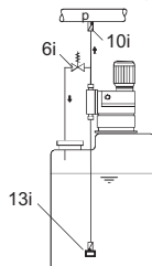
6-сур. Бакқа орнату
