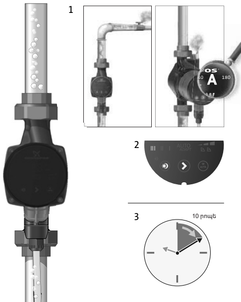
Նկար 13 Ջեռուցման համակարգերից օդի հեռացումը
