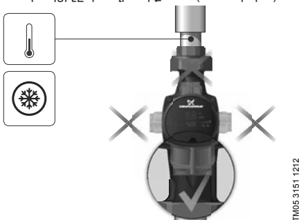
Նկար 6 Կառավարման բլոկի դիրքը պոմպի՝ օդորակման և U2 համակարգերում տեղադրման ժամանակ
