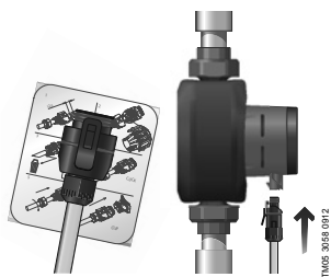
Рис. 10 Подключение к электросети
