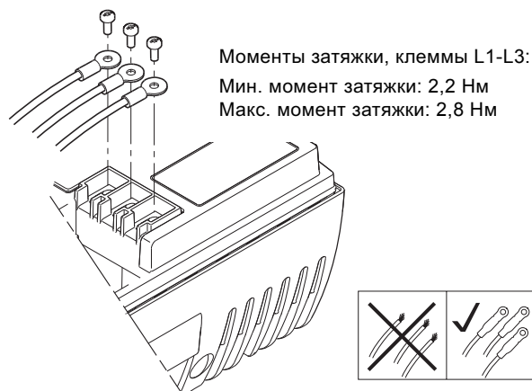
Рис. 5 Подключение электропитания
