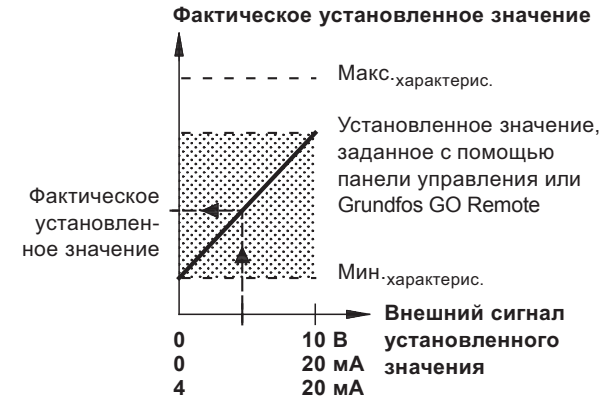
Рис. 23 Зависимость между фактическим установленным значением и внешним сигналом установленного значения в разомкнутой цепи регулируемого режима
