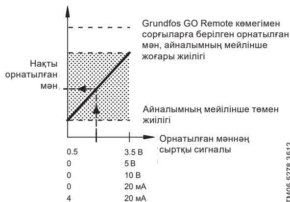
25-сур. Нақты орнатылған мән мен тұрақты сипаттама пайдалану кезіндегі орнатылған мәннің сыртқы сигналы арасындағы тәуелділік
