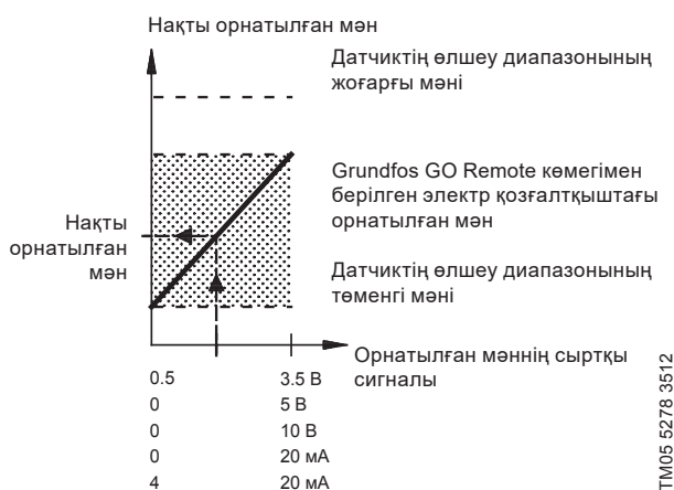
24-сур. Нақты орнатылған мән мен датчик бойынша кері байланыспен пайдалану кезіндегі орнатылған мәннің сыртқы сигналы арасындағы тәуелділік
