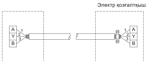
11-сур. 3 тарамды қоршалған кабельді қосу
