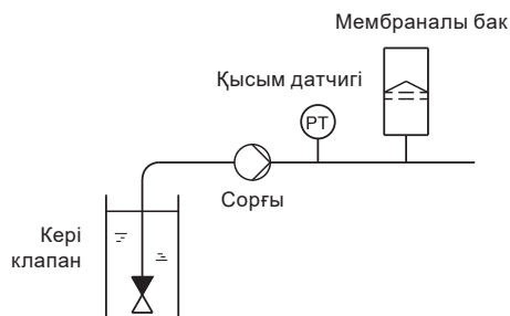
51-сур. Сорғыш жүйедегі кері клапан мен қысым датчигінің орны
