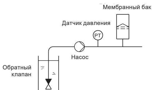
Рис. 51 Положение обратного клапана и датчика давления в системе с всасыванием
