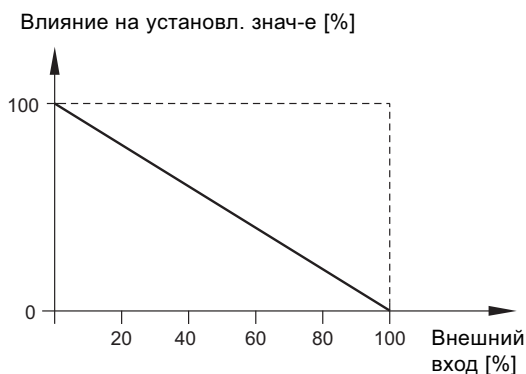
Рис. 45 Обратная функция
