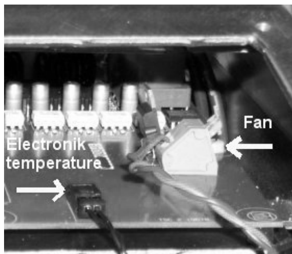
Рис. 20 Датчик контроля температуры в клеммной коробке
