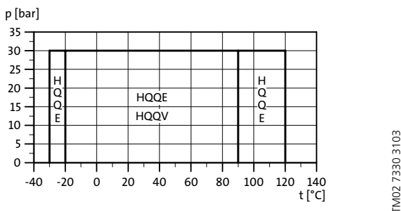
Рис. 14 Область эксплуатации стандартных уплотнений вала
