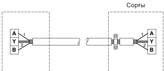
9-сур. 2 тармақты экрандалған кабельді жалғау
