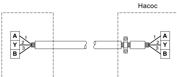
Рис. 8 Подключение 3-жильного экранированного кабеля
