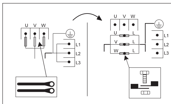
Рис. 25 Переключение насоса типа «Е» из нормального режима работы в аварийный
