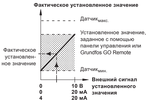
Рис. 22 Зависимость между фактическим установленным значением и внешним сигналом установленного значения в регулируемом режиме
