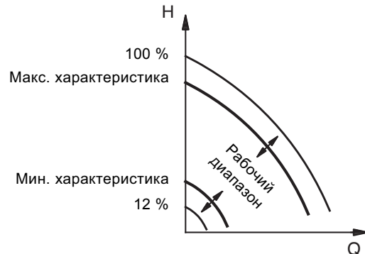
Рис. 20 Установка мин. и макс. характеристик в % от максимальной производительности
