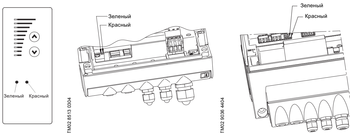
Рис. 24 Световые индикаторы на насосах с трёхфазными электродвигателями
