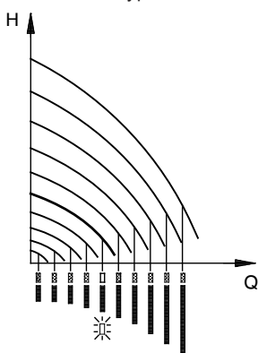
17-сур. Реттелмейтін режимдегі сорғы өндірімділігін баптау
