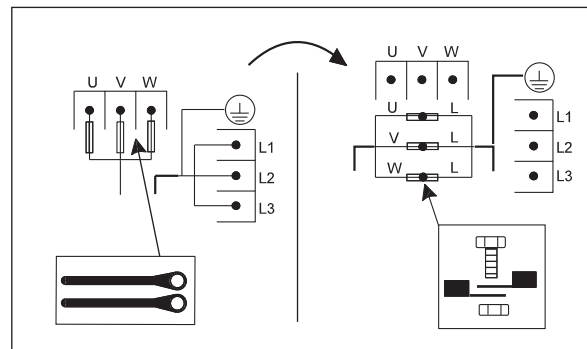
26-сур. «Е» типіндегі сорғының қалыпты жұмыс режимінен авариялыққа ауысуы
