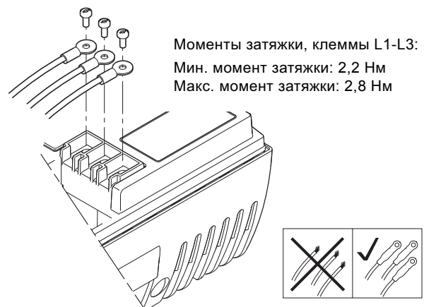
Рис. 5 Подключение электропитания
