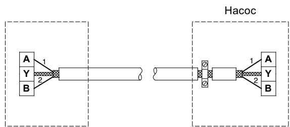
Рис. 9 Подключение 2-жильного экранированного кабеля
