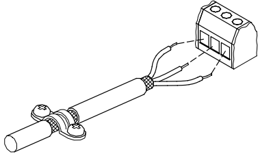
Рис. 7 Соединение оплетки и проводов экранированного кабеля с колодкой
