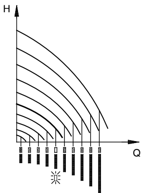
11-сур. Реттелмейтін режимдегі сорғы (тұрақты сипаттама)
