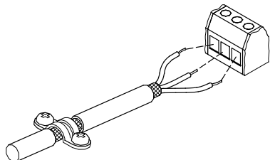
7-сур. Қалыпты экрандалған кабельдер орамы мен сымдарын қосу
