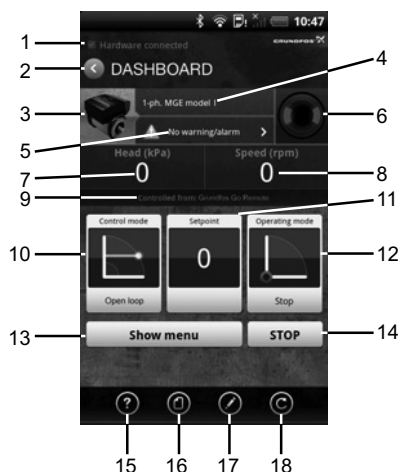
Рис. 19 Пример панели индикации
