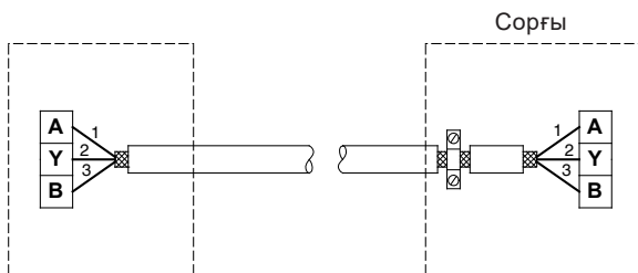
8-сур. 3 тармақты экрандалған кабельді жалғау
