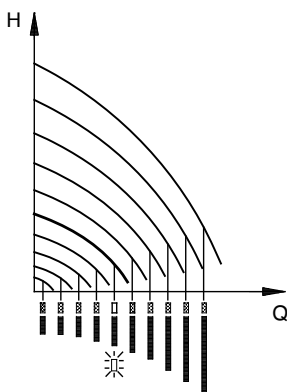
Рис. 17 Настройка производительности насоса в нерегулируемом режиме
