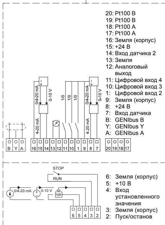
Рис. 6 Схема соединений
