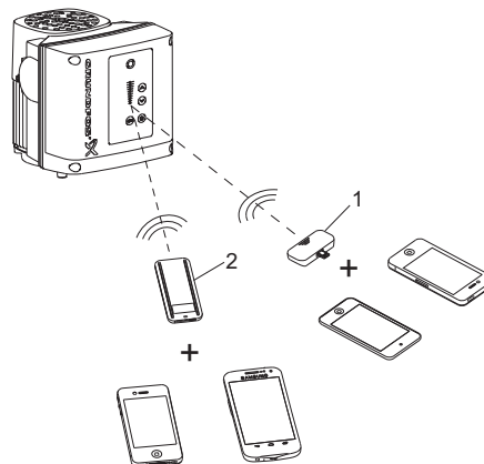
18-сурет. Инфрақызыл сигнал арқылы Grundfos GO Remote және сорғы арасындағы байланыс
