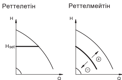
12-сур. Реттелетін (тұрақты қысым) немесе реттелмейтін (тұрақты сипаттама) режимдегі сорғы
