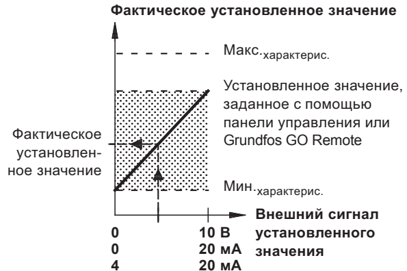
Рис. 23 Зависимость между фактическим установленным значением и внешним сигналом установленного значения в разомкнутой цепи регулируемого режима
