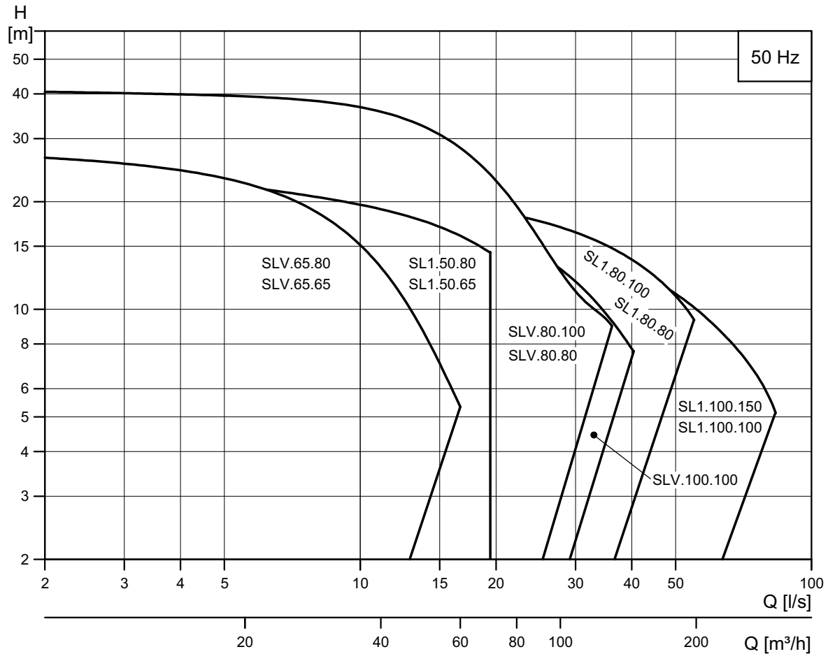
Рис. 3 Диапазон производительности
