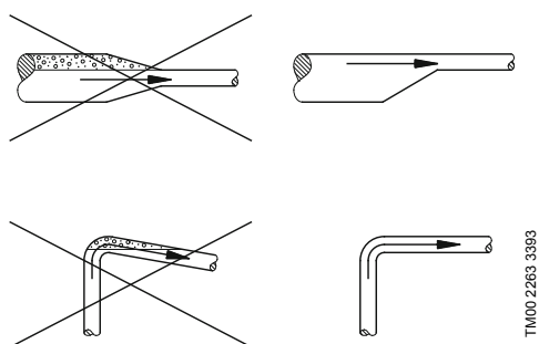
Рис. 22 Установка трубопроводов
