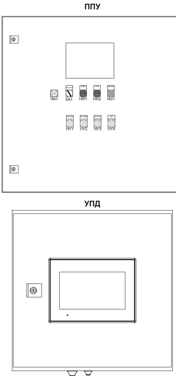
Рис. 8 Прибор управления пожарными насосами Control MX
