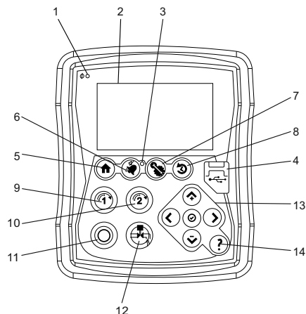
Рис. 12 Пользовательский интерфейс
