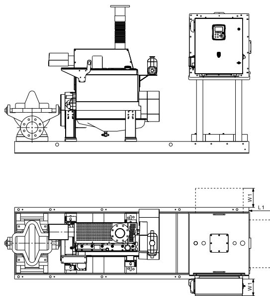
Рис. 2 Насосная установка, вид слева и сверху
