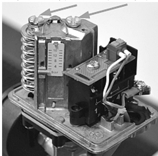
9-сур. FRG-2 қысым релесін баптау
