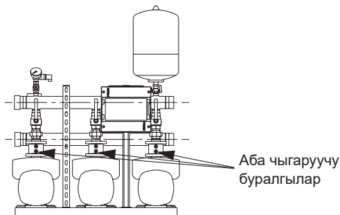
7-сүр. СМЕ-А/-I соркысмалары менен тутумдарда аба чыгаргыч буралгылардын жайгашуусу
