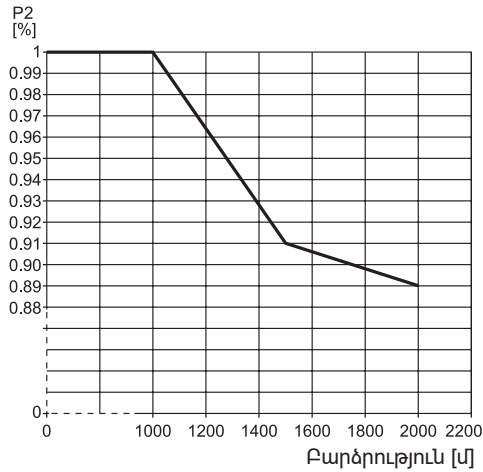
Նկար 20 Էլեկտրաշարժիչի ելքային հզորության (P2) նվազումը կախված ծովի մակերևույթի նկատմամբ բարձրությունից:
