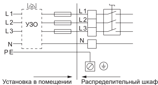
Рис. 5 Пример подключения Hydro Multi-E к сети с защитными предохранителями и дополнительной защитой (применимо только к системам с однофазными электродвигателями)
