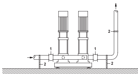
4-сур. Құбырларды діріл қосылуы мен тіреуіштерімен бірге орнатудың мысалы
