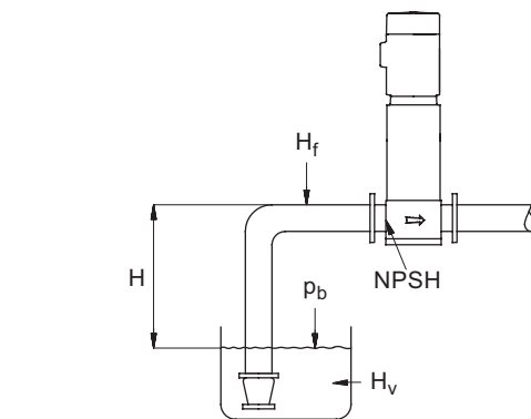
Նկար 21 Բարձրացման նվազագույն ճնշման հաշվարկի համար անհրաժեշտ պարամետրերը
