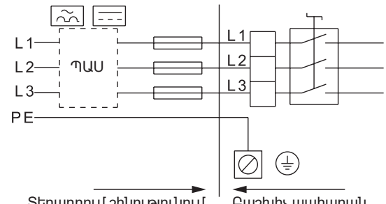
Նկար 6 Hydro Multi-E-ի պաշտպանիչ ապահովիչներով և լրացուցիչ պաշտպանությունով համալրված ցանցին միացման օրինակ (կիրառելի է միայն եռաֆազ էլեկտրաշարժիչներով համակարգերի համար)
