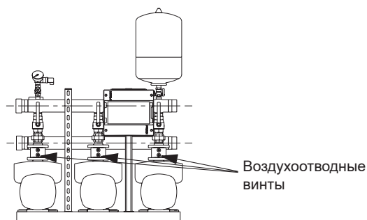
Рис. 7 Расположение воздухоотводных винтов в системе с насосами SME-A/-I
