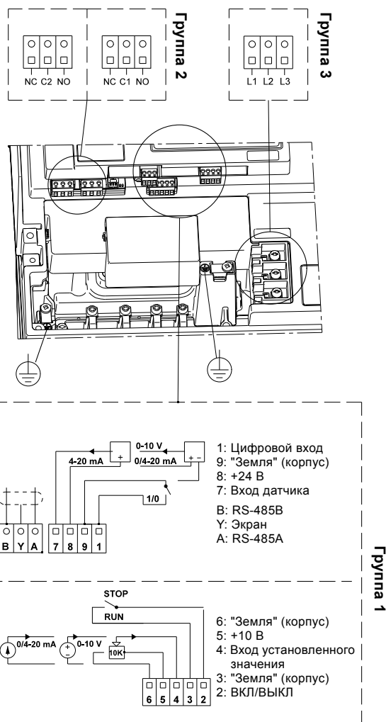
Рис. 14 Клеммы насосов TPE, NKE, NKGE и NBE, NBGE
