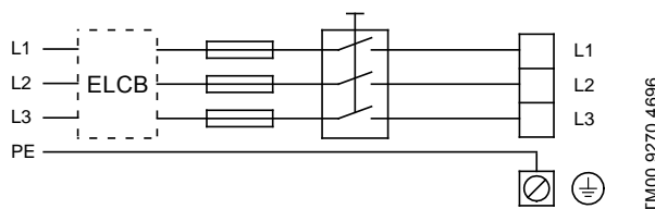
Рис. 6 Подключенный к сети насос с сетевым выключателем, плавкими предохранителями, дополнительной защитой и защитным заземлением
