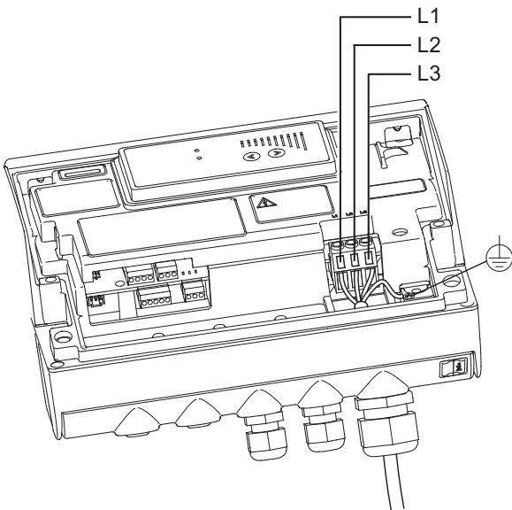
Рис. 7 Подключение электропитания
