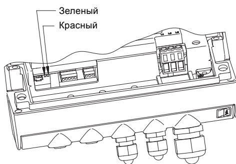
Рис. 37 Световые индикаторы на насосах с однофазными электродвигателями
