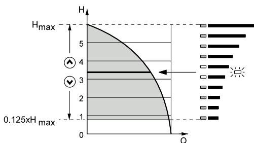
Рис. 27 Установленное значение задано равным 3,4 м (регулирование по разности давлений)
