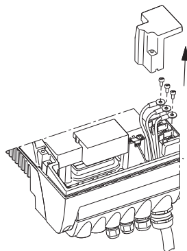
Рис. 30 Отключение силовых проводов
