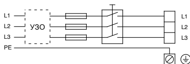
Сүрөт 2 Түйүнгө туташтырылган насос тармактык ажыркычы, тез эрип кетүүчү сактагыч, кошумча коргоо жана коргоочу жердетүү менен
