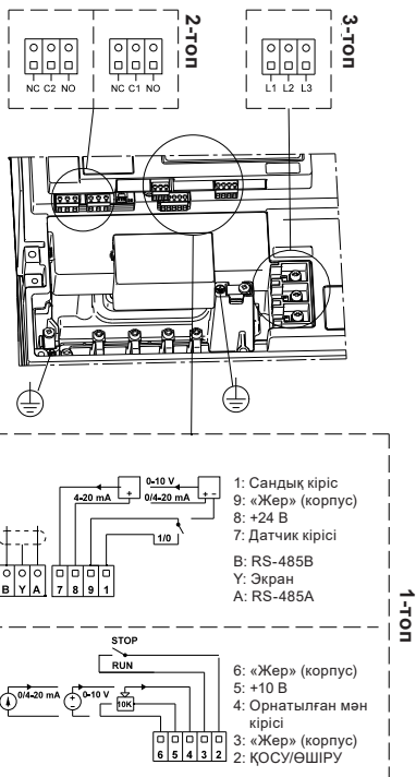
6-сур. TPE, NKE, NKGE және NBE, NBGE сорғыларының клеммалары
