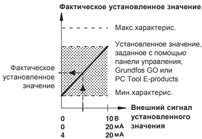
Рис. 28 Зависимость между фактическим установленным значением и внешним сигналом установленного значения в разомкнутой цепи регулируемого режима
