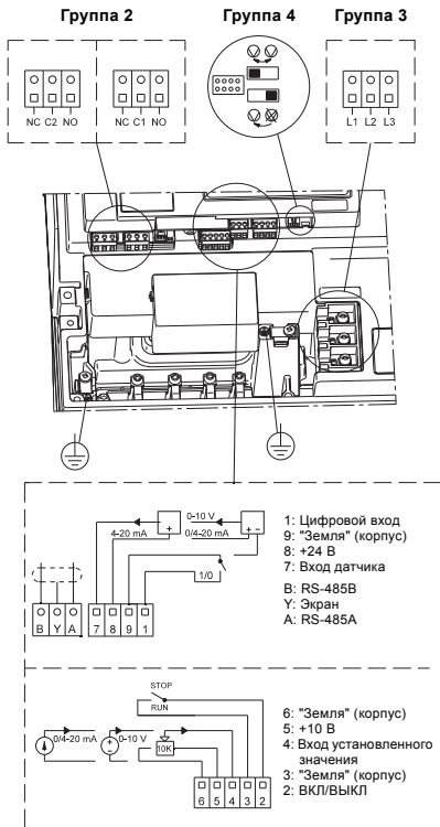
Рис. 7 Клеммы насосов TRPED
