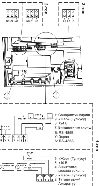
Сүрөт 6 Насостор клеммасы TPE, NKE, NKGE жана NBE, NBGE
