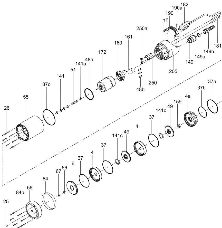
Рис. 1 SB pump
