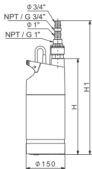
Рис. 11 Насос SB. Одинаковые размеры исполнений со встроенным и исполнений с плавучим сетчатым фильтром впускного патрубка
