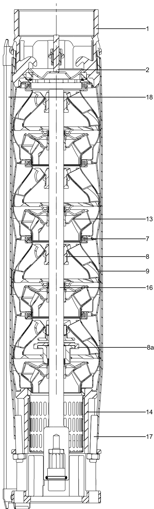
Рис. 10 Пример SP 46
