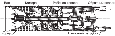
Рис. 1 Вид насосов SQ и SQE без электродвигателя
