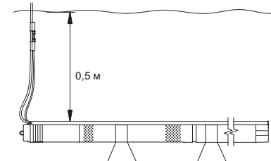
8-сур. Көлденең күйіндегі орнатылым
