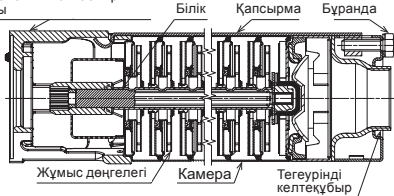
2-сур. Электр қозғалтқышсыз сыртқа тебу орындалымындағы SQF сорғыларының түрі.
