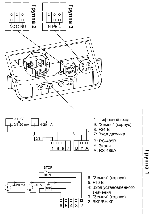
Рис. 4 Клеммы насосов TPE серии 2000
