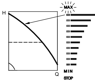
Рис. 33 Макс. характеристика
