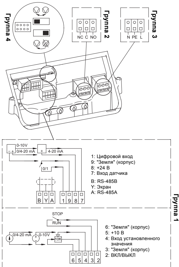
Рис. 5 Клеммы насосов TPED серии 2000
