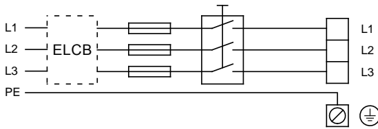
Рис. 6 Подключенный к сети насос с сетевым выключателем, плавкими предохранителями, дополнительной защитой и защитным заземлением
