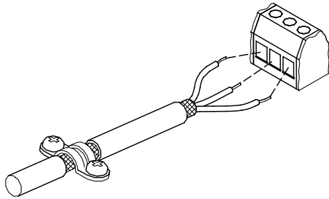
Рис. 11 Зачищенный кабель с экраном и проводными соединениями
