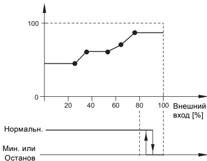
Рис. 63 Таблица влияни. с остан. у макс.
