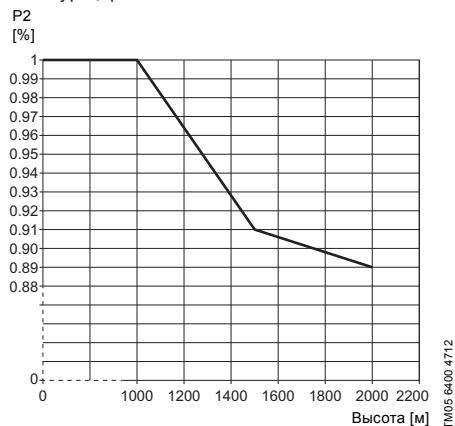
29-сур. Теңіз деңгейінен жоғары биіктікке байланысты электр қозғалтқыштың (P2) шығару қуаттылығының төмендеуі
