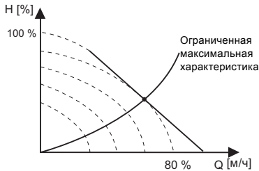
53-сур. Ең жоғарғы сипаттамаға әсерін тигізетін қуаттылық пен қысымға шектеулер
