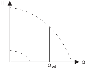
Рис. 48 Постоянный расход
