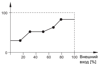
Влияние на установл. знач-е [%]
