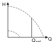
Тұрақты шығын
