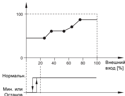
Влияние на установл. знач-е [%]
