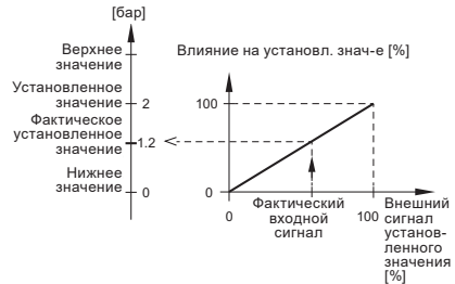
Рис. 56 Пример настройки регулирования установленного значения
