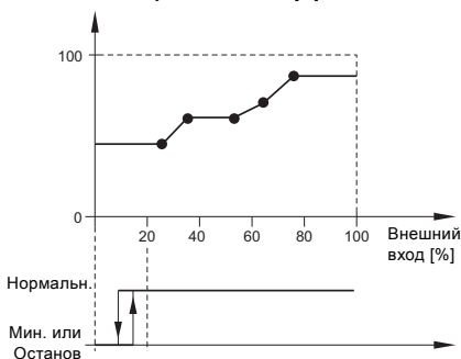
Рис. 62 Таблица влияни. с остан. у мин.
