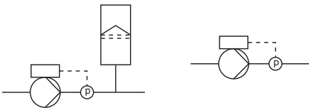
Рис. 41 Постоянное давление
