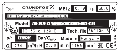
5-сур. TP, TPD жарылысқа қорғалған сорғыларының фирмалық тақташасының үлгісі
