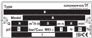
Рис. 4 Образец фирменной таблички насосов TP, TPD, TPE, TPED
