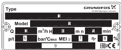
4-сур. TP, TPD, TPE, TPED сорғыларының фирмалық тақташасының үлгісі
