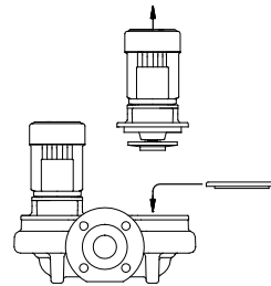
Рис. 22 Установка глухого фланца
