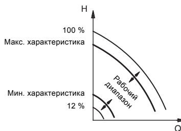
Рис. 25 Установка мин. и макс. характеристик в % от максимальной производительности
