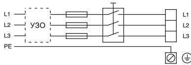
Նկար 2 Ցանցին միացված պոմպը ցանցային անջատիչով, դյուրահալ ապահովիչներով, լրացուցիչ պաշտպանությամբ և պաշտպանիչ հողանցումով
