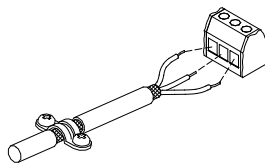
Նկար 8 Վահանավորվախ մալուխի հյուսապատվածքի և հարողաարերի միացումը կադապարին
