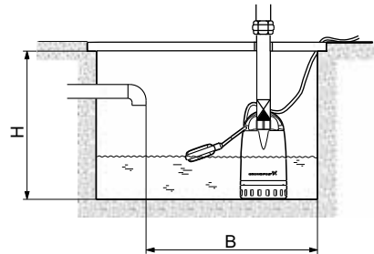
Նկար 3 Նվազագույն մոնտաժային չափեր
