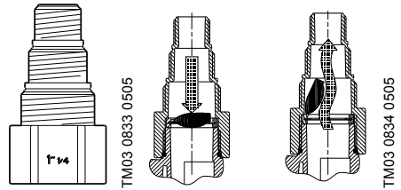
Նկար 6 Հարմարակցիչ և հետադարձ կապույր (դիրք և գործառույթ)
