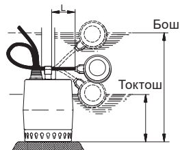
7-сүр. Коё берүү/токтотуу деңгээлдери, Unilift KP-A
