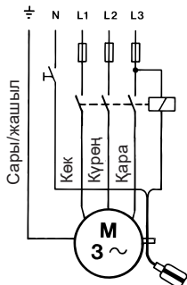
9-сүр. Электрдик туташуулардын схемасы
