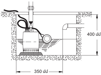
Նկար 3 Unilift KP-A համար հորի նվազագույն չափերը
