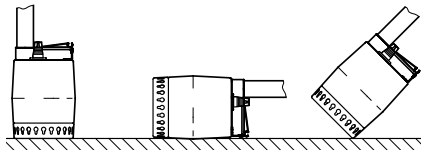
Рис. 5 Размещение Unilift KP-A и Unilift KP-M
