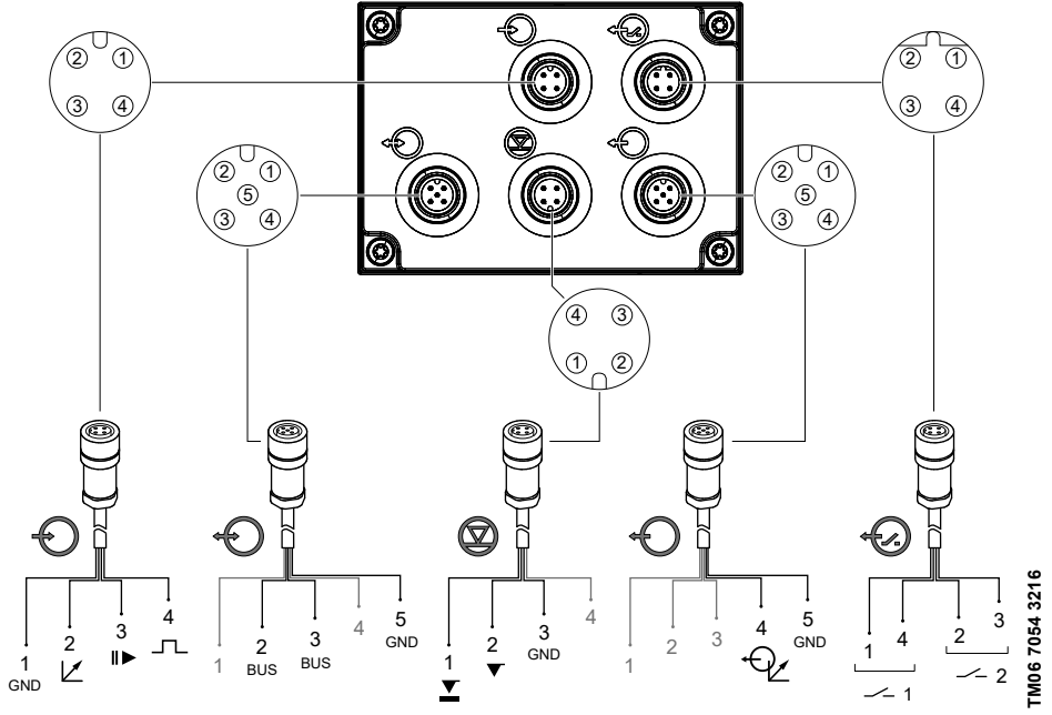
11-сур. Электр қосылыстардың схемасы
