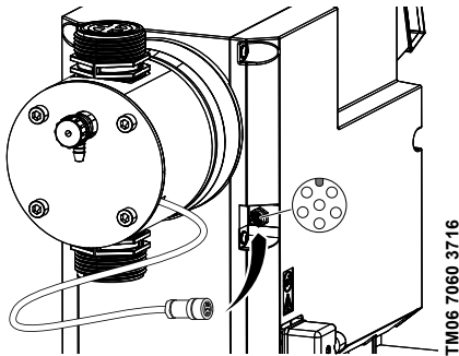
12-сур. FlowControl сигналының қосылуы
