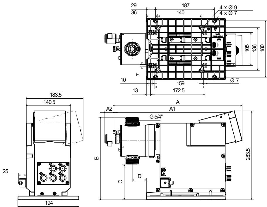
Рис. 43 Габаритный чертёж
