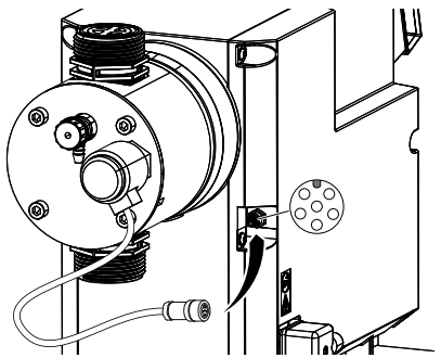
13-сур. ДРМ сигналының қосылуы
