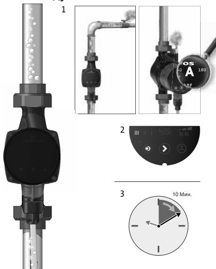
Рис. 13 Удаление воздуха из систем отопления
