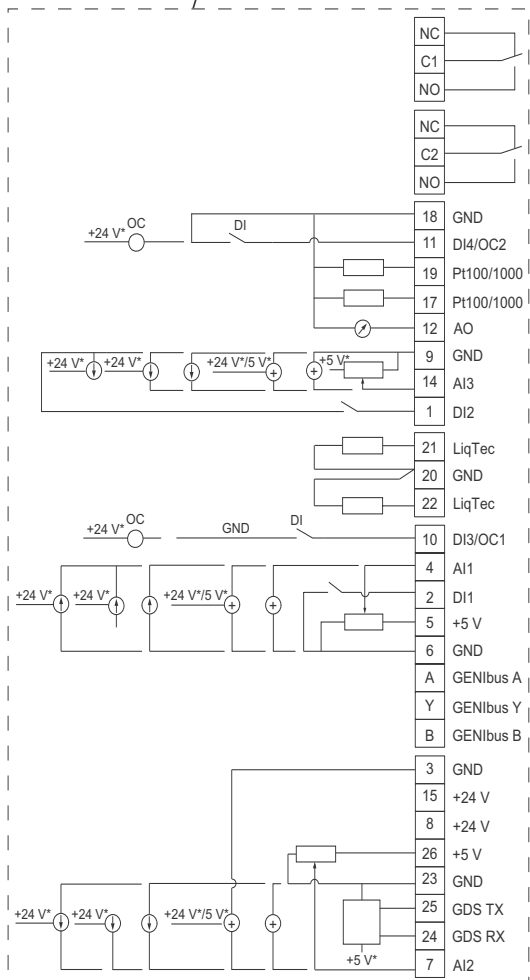
Рис. 8 Клеммы соединений, насосы CRE, CRIE, CRNE, SPKE и MTR
