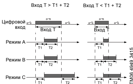
Рис. 43 Функция таймера длительности для цифровых входов
