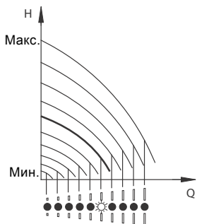
Рис. 19 Насос в режиме управления с постоянной характеристикой
