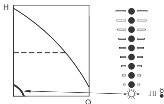
Рис. 21 Эксплуатация при минимальной характеристике
