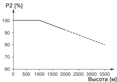
Рис. 14 Мощность электродвигателя в зависимости от высоты над уровнем моря
