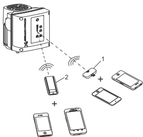
Рис. 24 Связь между Grundfos GO и насосом посредством радио- или инфракрасного сигнала
