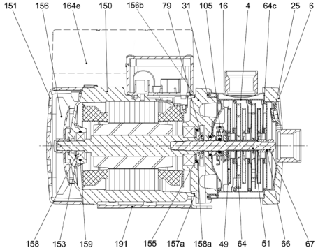
Նկար 2 CME պոմպի կտրվածքը
