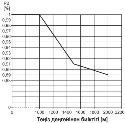
8-сур. P2 атаулы шығыс қуатының теңіз деңгейінің биіктігіне тәуелділігі
