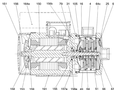
2-сур. СМЕ сорғысының кесігі
