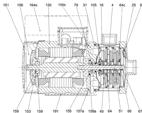
Рис. 2 Разрез насоса СМЕ
