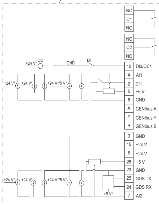
Рис. 9 Клеммы соединений, насос СМЕ
