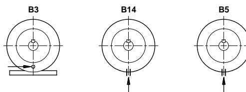
Рис. 3 Сливные отверстия
