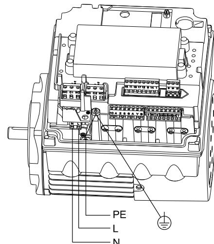
Рис. 5 Подключение к сети однофазных электродвигателей
