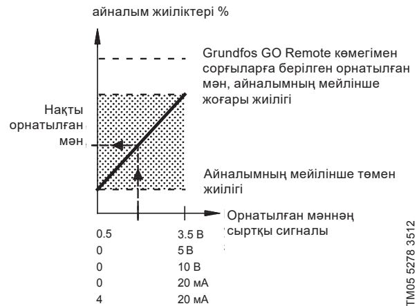
25-сур. Нақты орнатылған мән мен тұрақты сипаттама пайдалану кезіндегі орнатылған мәнің сыртқы сигналы арасындағы тәуелділік
