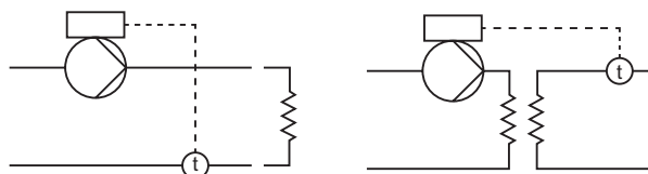
Рис. 30 Постоянная температура
