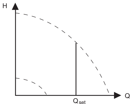
Рис. 38 Постоянный расход
