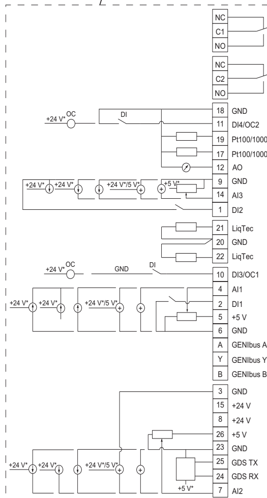
8-сур. Қосылыстар клеммалары, CRE, CRIE, CRNE, CRTE және MTRE сорғылары
