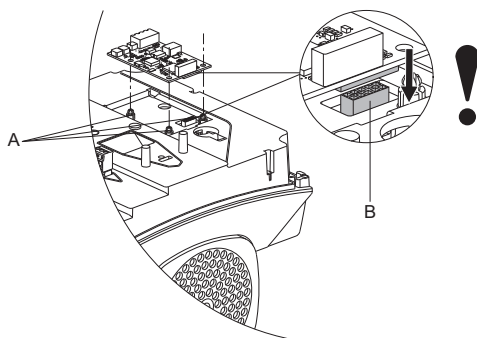
60-сур. СИМ модулін пластик ұстағыштар (А орны) деңгейімен бірдей орнатып, коннекторды (В орны) қосыңыз
