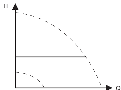
31-сур. Тұрақты қысым өзгерісі
