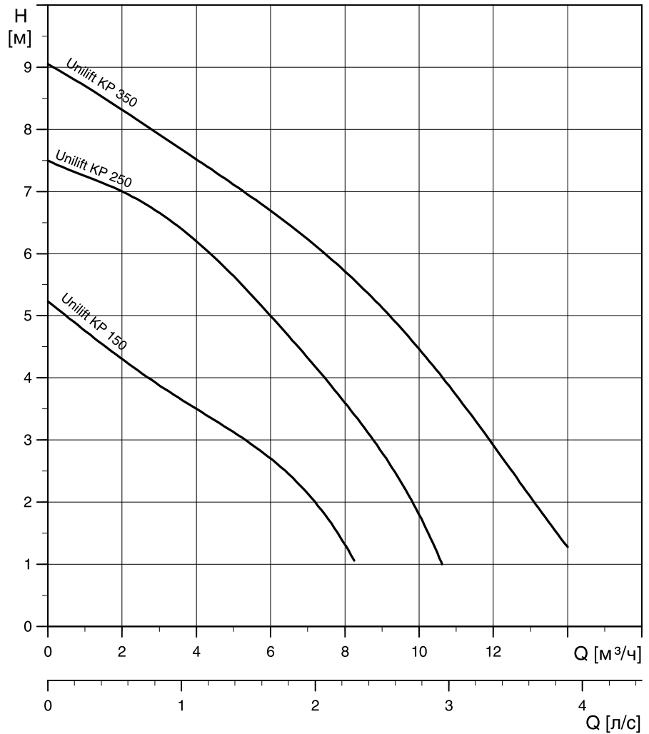
Рис. 7. Кривая характеристик
