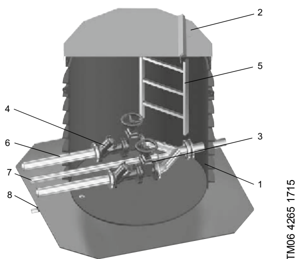
Рис. 129. Камера переключения
