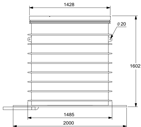
Рис. 132. Камера переключения, высота 1,6 м
