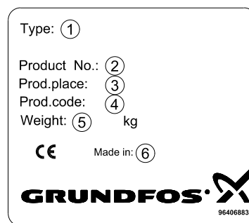
Рис. 2 Фирменная табличка
