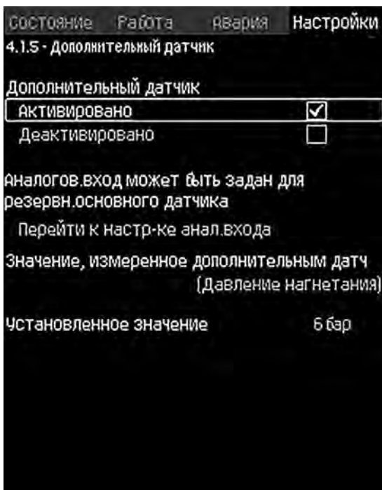
Меню настройки вспомогательного датчика.
