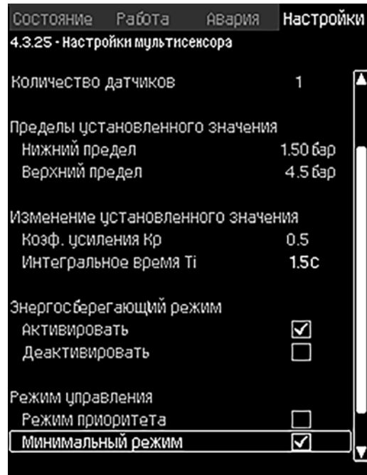
Главное меню режима работы с несколькими датчиками
