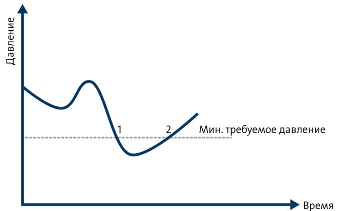
Если давление на одном или нескольких датчиках ниже требуемого заданного значения, установка повышения давления увеличивает производительность до тех пор, пока не будет превышено предельное значение на всех датчиках.
