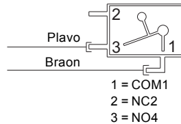
Slika 1 Dijagram ožičavanja
