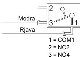
Slika 1 Shema ožičenja
