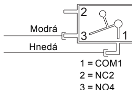
Obr. 1 Schéma zapojenia
