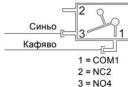
Фиг. 1 Схема на свързване
