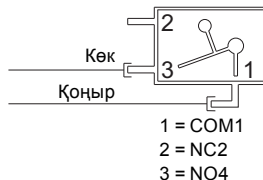
1. сур. Сымдық диаграмма
