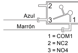
Fig. 1 Esquema de conexiones eléctricas
