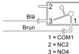
Fig. 1 Forbindelsesdiagram
