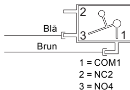
Fig. 1 Kopplingsschema
