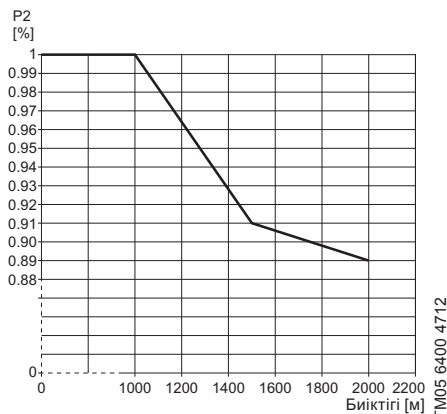
13-сурет Теңіз деңгейінен жоғары биіктігіне байланысты электр қозғалтқыштың (P2) шығыс қуатын төмендету
