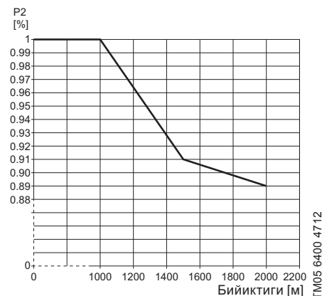
13-сүр. Электр кыймылдаткычынын чыгуу кубаттуулугунун деңиз деңгээлинен бийиктигине жараша төмөндөөсү (P2)
