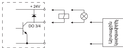
Նկար 41 Կարգավորվող թվային մուտքերի և ելքերի օրինակ
