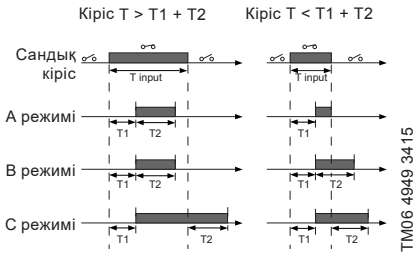
40-сурет Сандық кірістердің ұзақтық таймерінің функциясы
