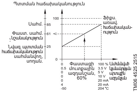
Նկար 45 Մշտական բևեռագրով սահմանված նշանակության կարգավորման օրինակ
