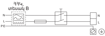
Նկար 4 Էլեկտրասնուցման անջատիչով, դյուրահալ ապահովիչնով և լրացուցիչ պաշտպանությամբ ապահովված էլեկտրական շարժիչը ցանցին միանալու օրինակ
