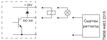
41-сурет Теңшелмелі сандық кірістер немесе шығыстар мысалы
