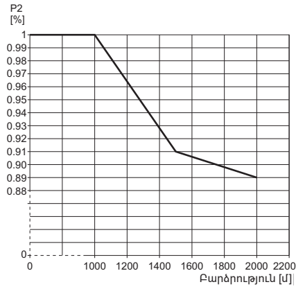
Նկար 13 Էլեկտրական շարժիչի (P2) ելքային հզորության նվազում՝ կախված բարձրությունից ծովի մակարդակից:
