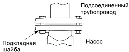
Рис. 5 Использование шайб для овальных отверстий под болты
