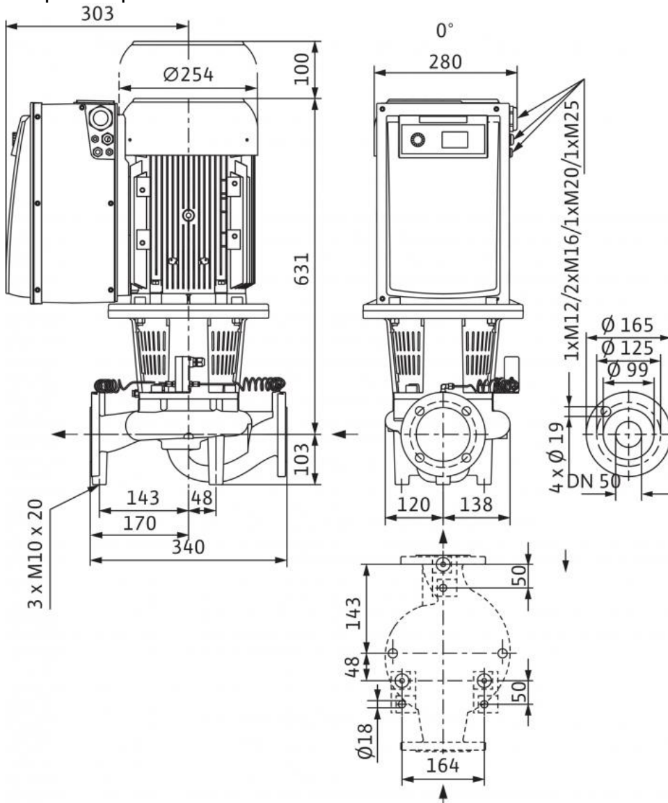
Габаритный чертёж
