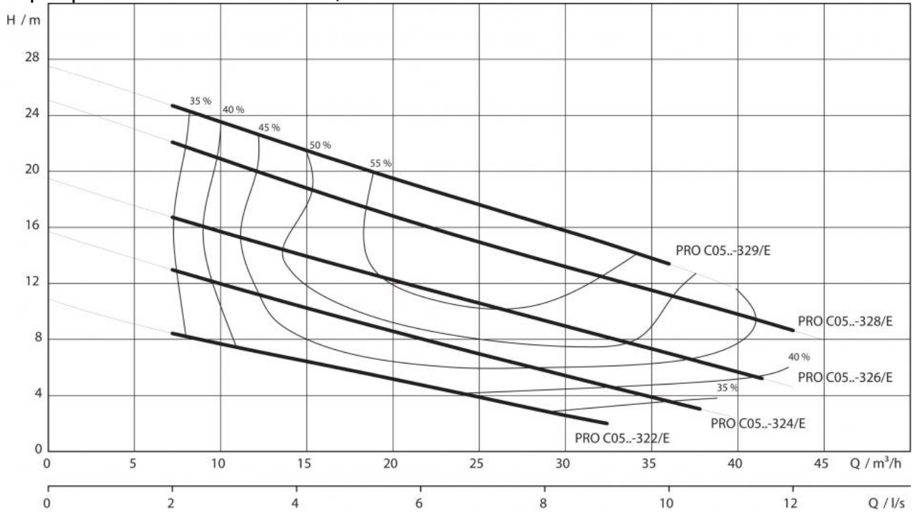
Характеристики Wilo-Rexa PRO V05.. - 50 Гц - 2900 об/мин
