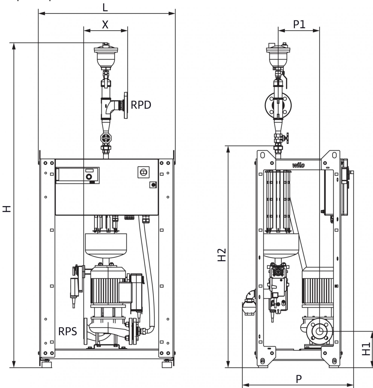
Габаритный чертеж
