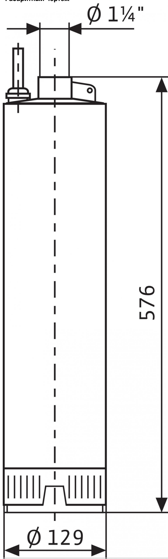
Габаритный чертеж
