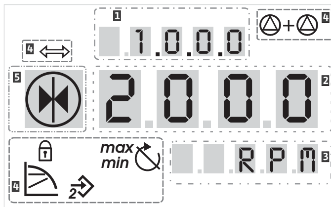
Рис. 30: Структура дисплея
