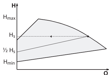
Рис. 11: Регулирование Др-в
