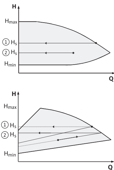
Рис. 43: Регулирование Др-с/Др-в
