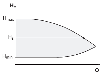
Рис. 10: Регулирование Др-с
