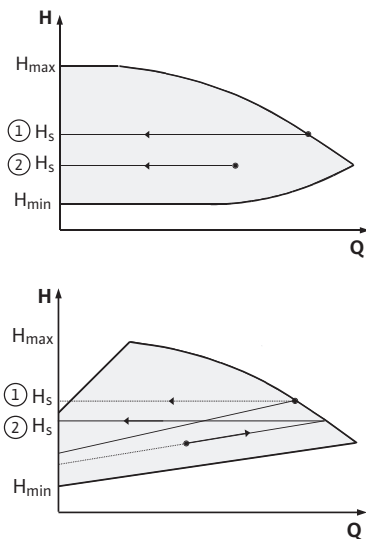
Рис. 43: Регулирование Δp-с/Δp-v
