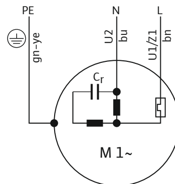
Fig. 8: Схема подсоединения однофазного электродвигателя
