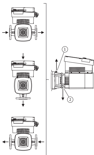
Fig. 23: Допустимые варианты монтажа с горизонтальным валом электродвигателя
