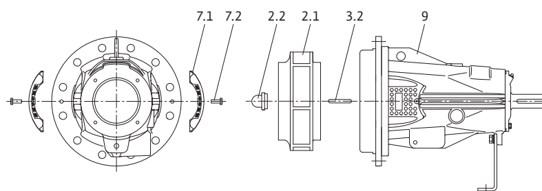
Fig. 25: Вставной блок
